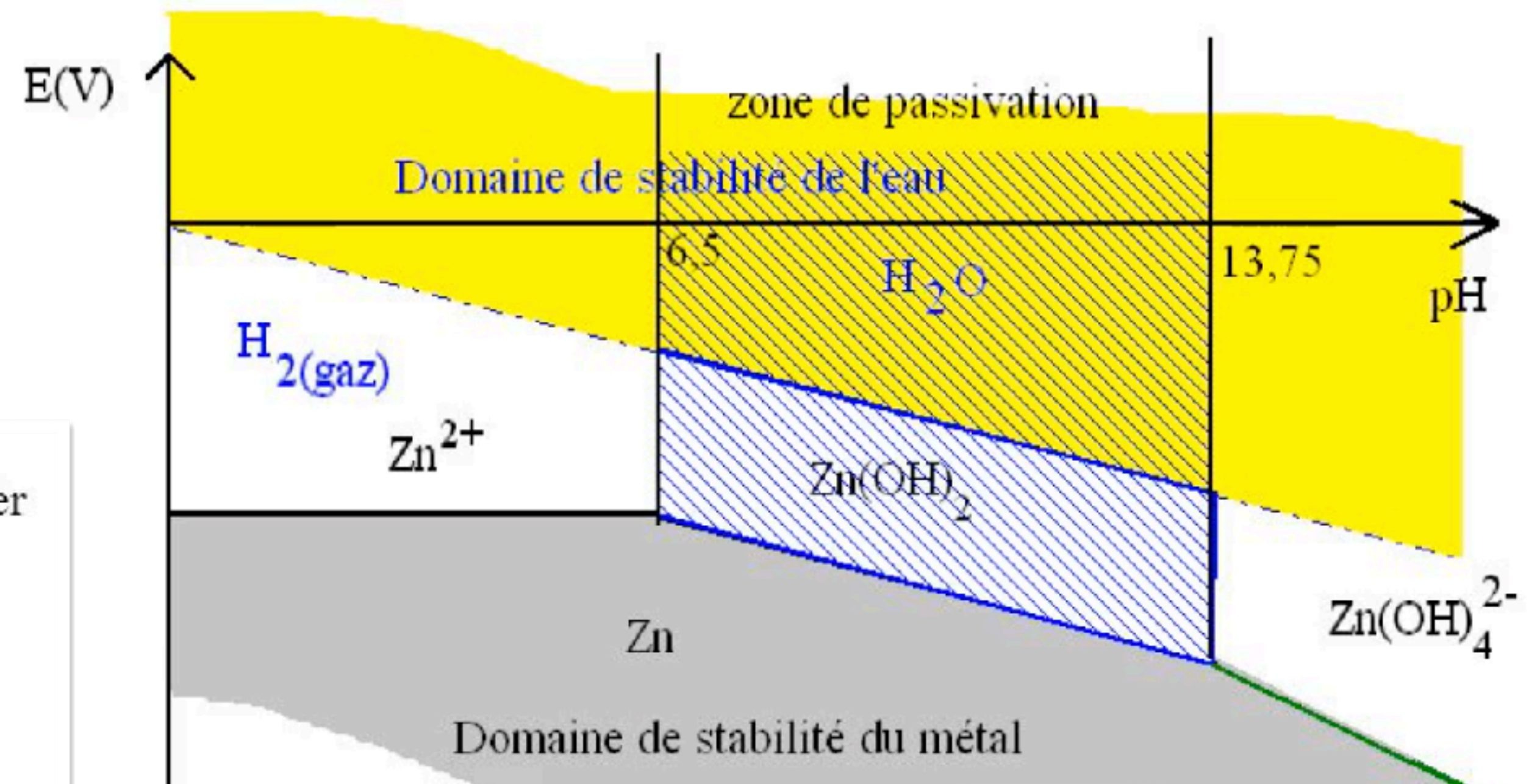
Diagramme potentiel-pH du zinc
